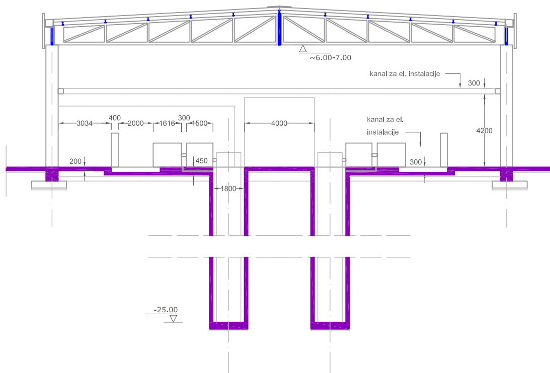
Presek 1-1
